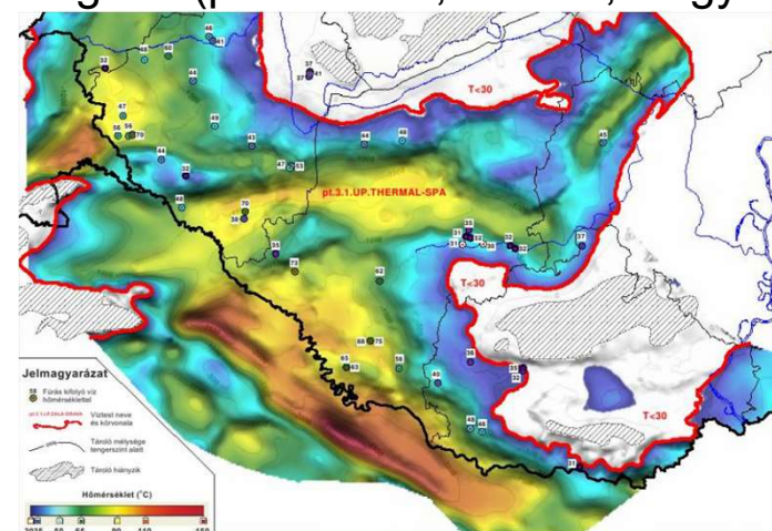
A Felső-Pannon termálvízadó réteg hőmérsékleti viszonyai Forrás: A Dráva-medence geotermikus erőforrásainak értékelése, DravaGeo projekt, 2012
